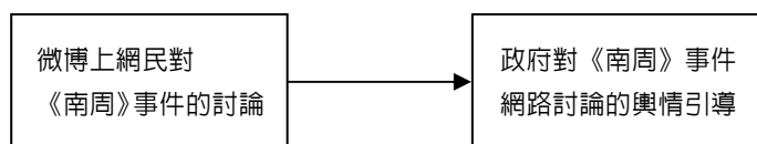
圖 1 研究架構圖
